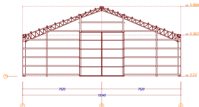
Giebelansichten
