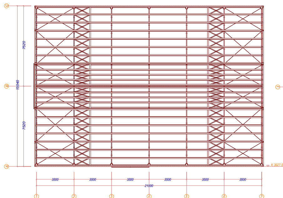
Draufsicht
