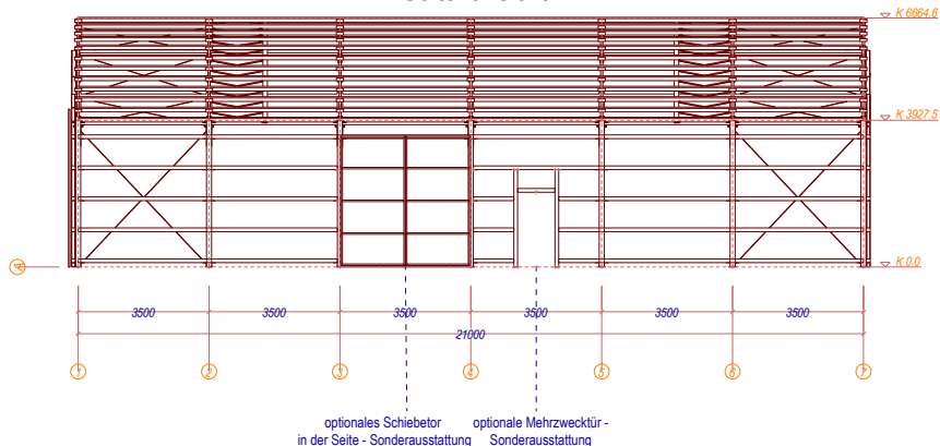
Seitenansicht
